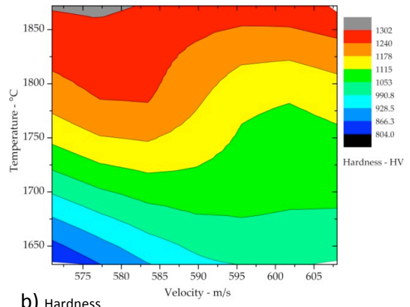
b) Hardness
