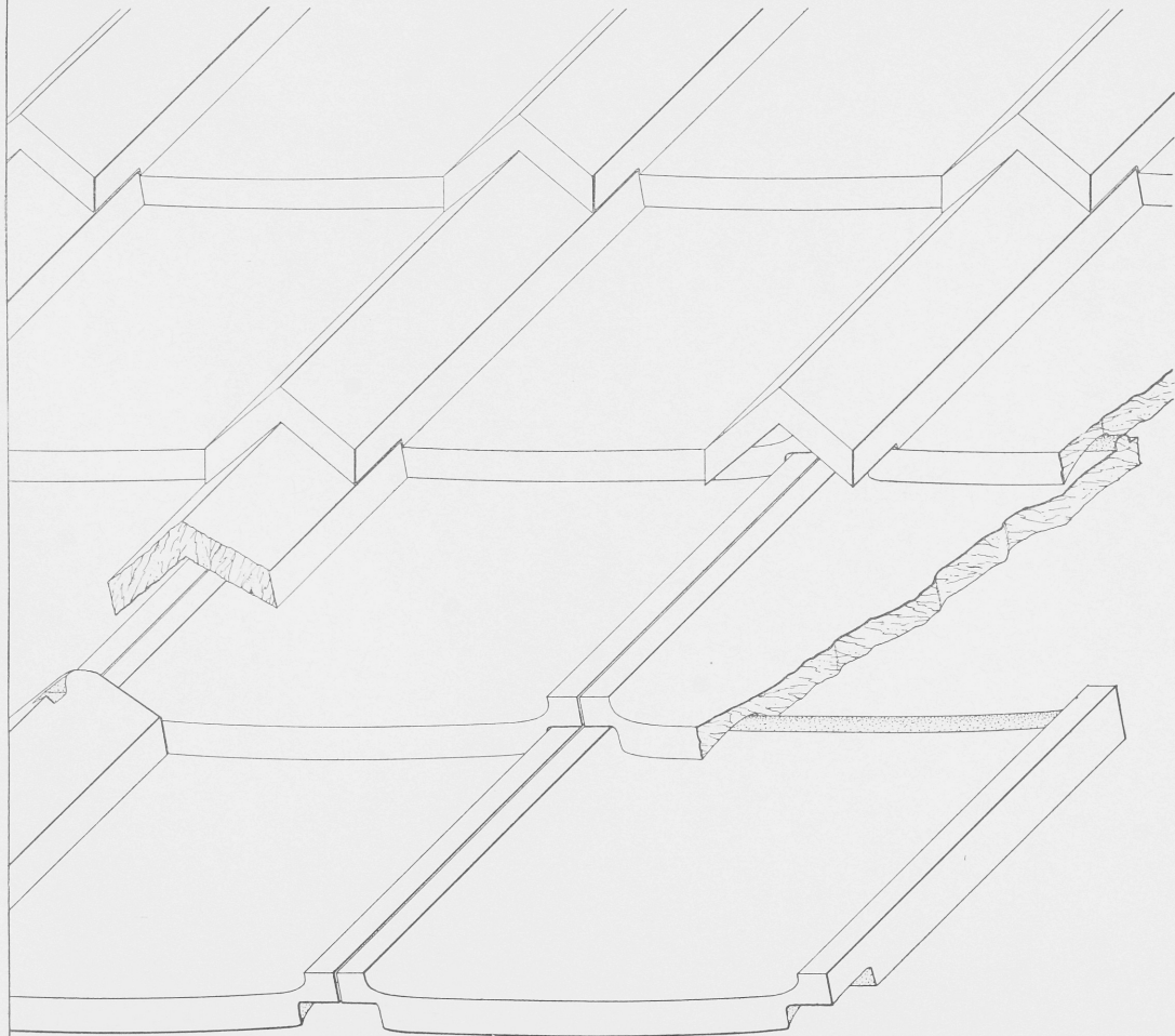
TEGVLA SCALE 1:6
